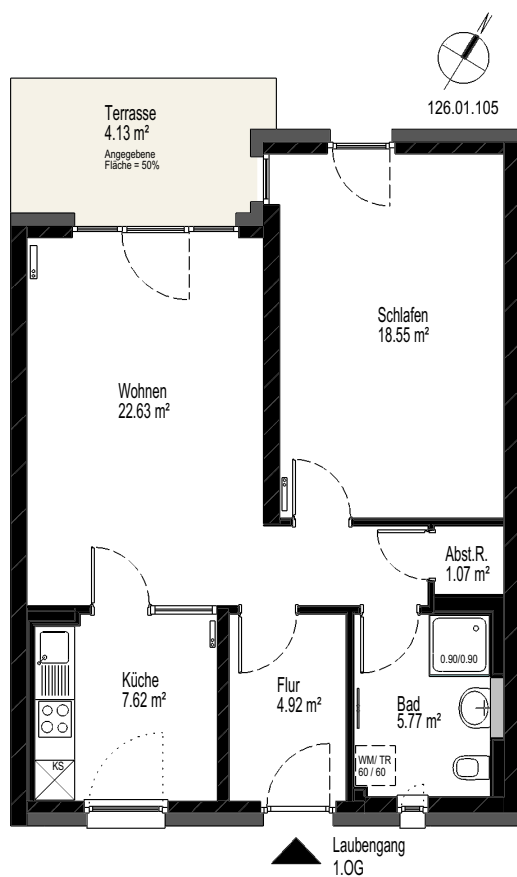
z. B. 2-Zimmer-Wohnung im 1. Obergeschoss, ca. 63 m 2
