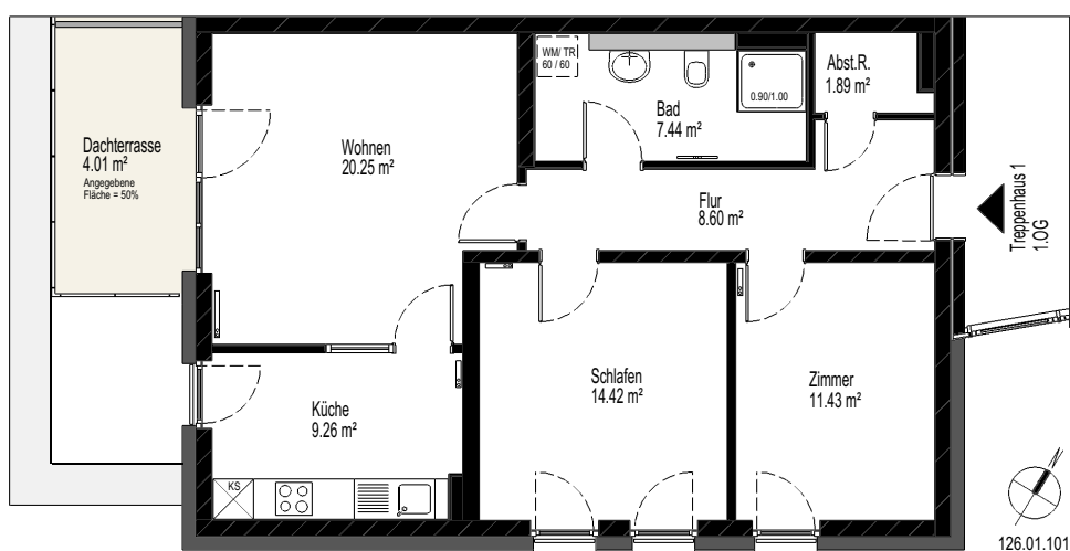
z. B. 3-Zimmer-Wohnung im 1. Obergeschoss, ca. 75 m 2
